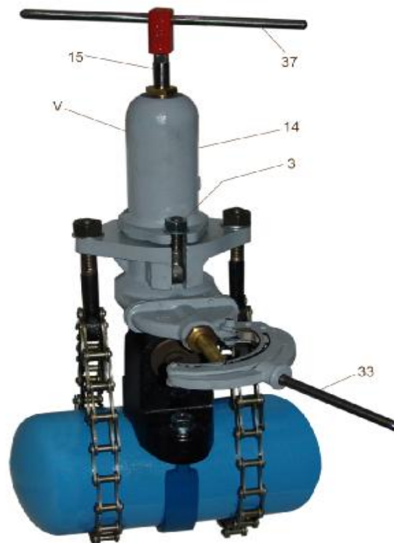
Abb. 3: Ventileinführung
